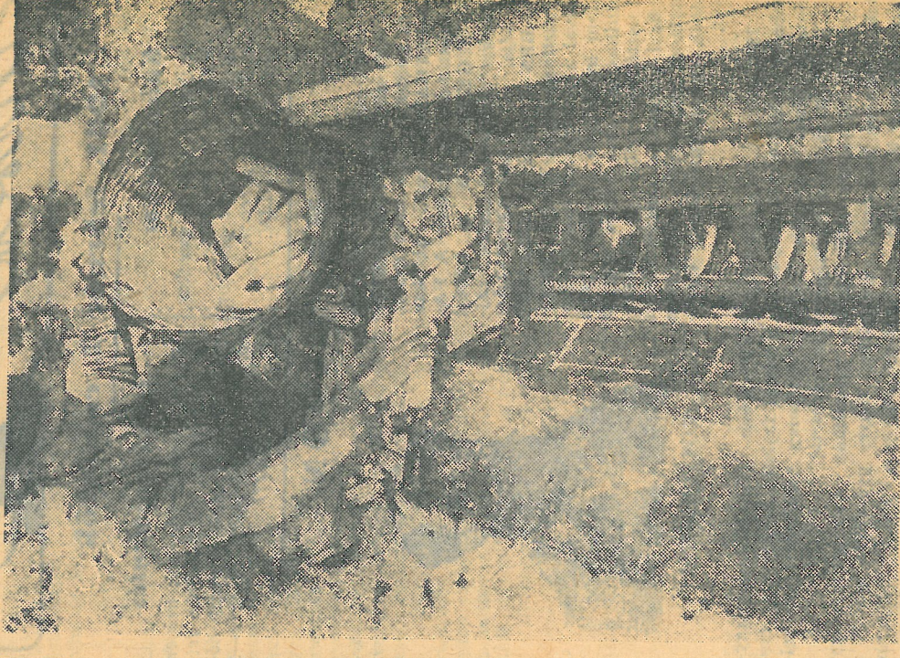
Néhány ügyes ötlettel kukoricamorzsolásra alakították át egy cséplőgépet a vaszari termelőségvetkezeti újtói. Ez a kép az átalakított gépet ábrázolja. Munka közben természetesen a két oldalt leharasztó fedőlemezt visszahajlítják, hogy a szétpattingo kukoricaszemek kárba ne vesszenek.
