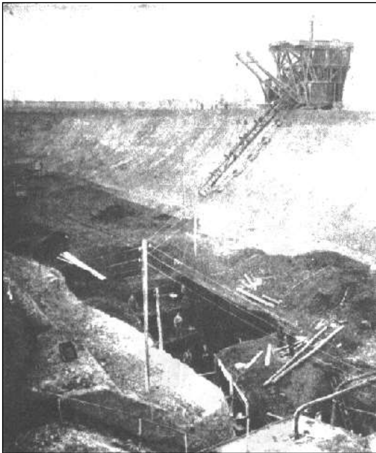
A Hungária külfejtés az 1910-es években. A fedőréteg eltávolítására használt serleges mélybagger. A 95 tonna súlyú gőzhajtású gép 13,5 m vastag földréteg eltávolítására volt alkalmas.
